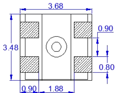
建议焊盘图
