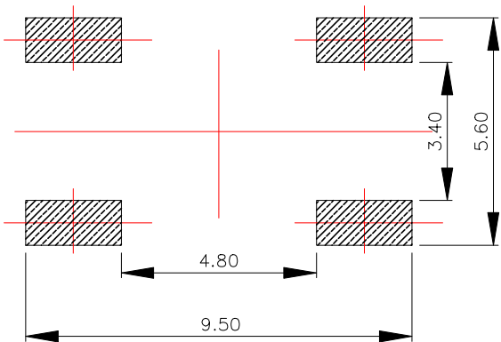
PCB. 焊接图
