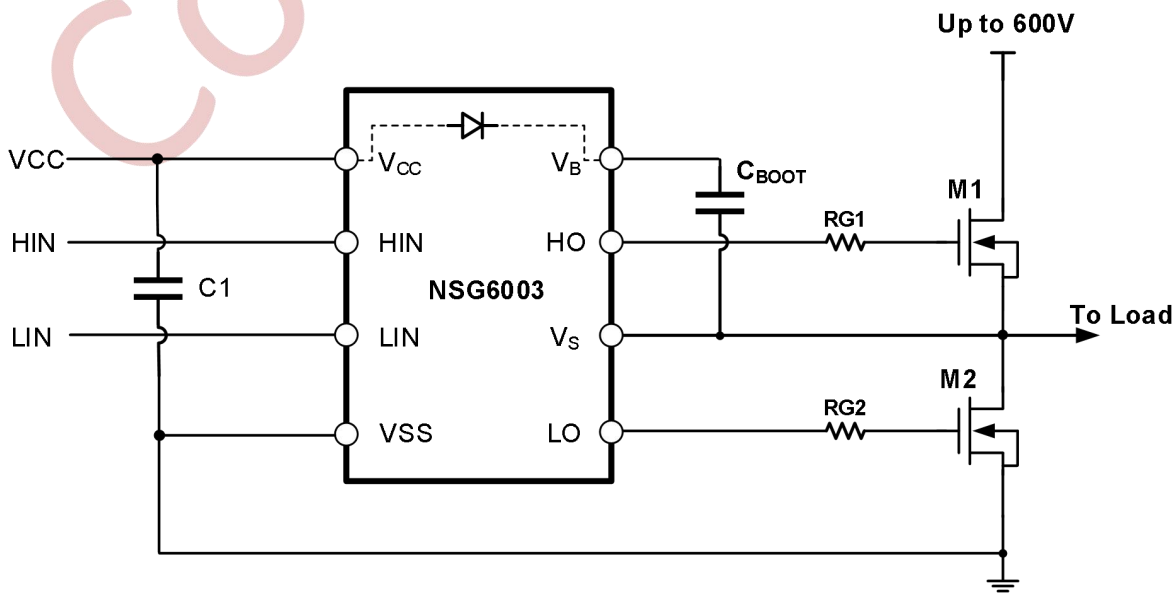
图 10-2 NSG6003 典型应用电路图
