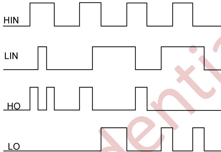
图 9-1 NSG6003 输入输出时序波形
