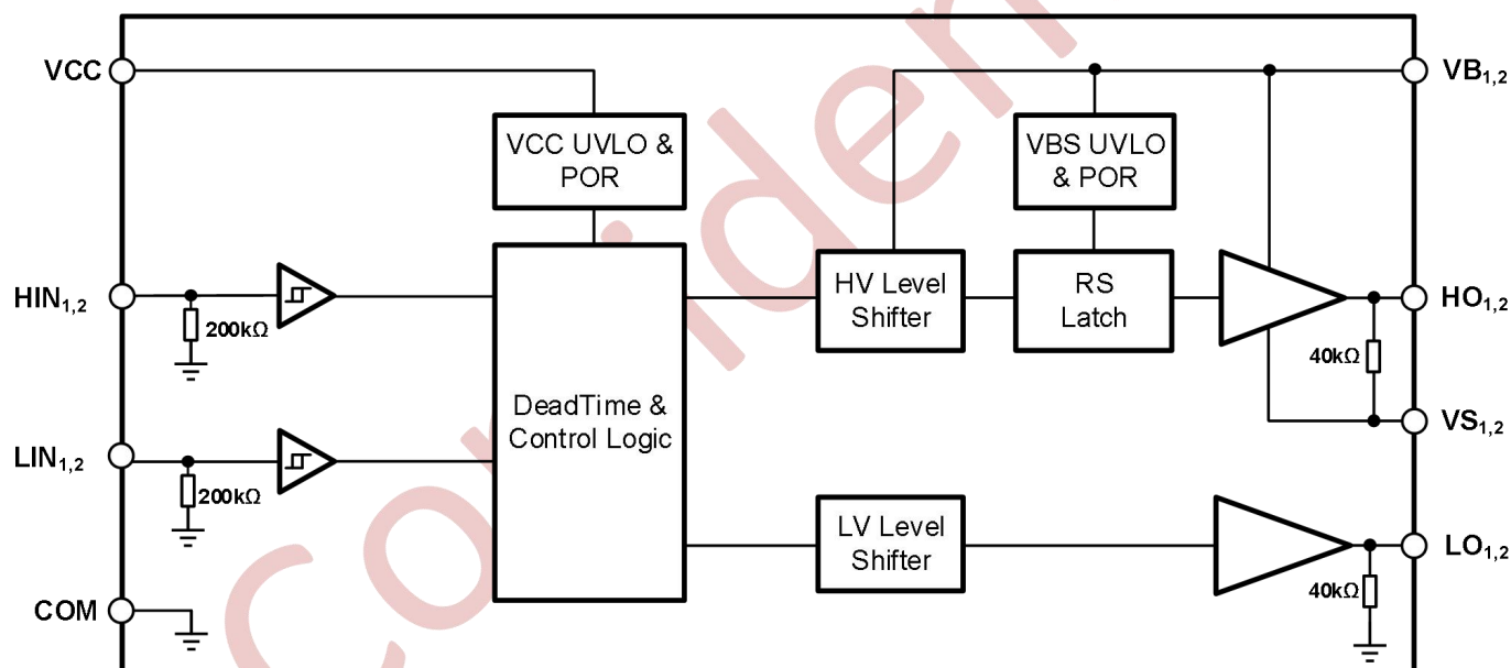
图 10-1 NSG1040 功能框图
