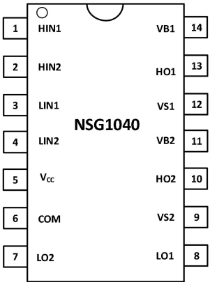
图 7-1 14-脚 SOP 顶视图
