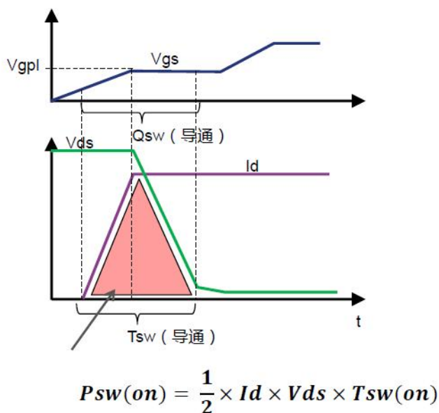
图 11-3 阻性负载条件下的 MOS 开关损耗
