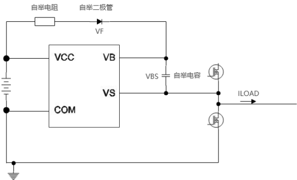
图 11-2 自举电路基本结构
