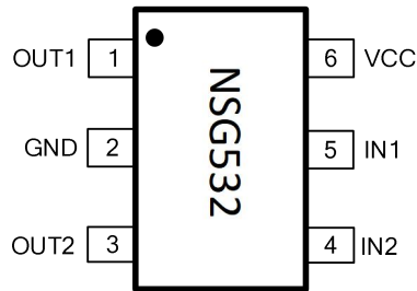
图 7-1 6-脚 SOT23-6 顶视图
