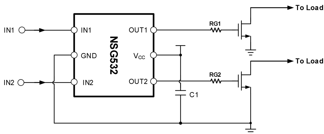
图 11-1 NSG532 典型应用电路图
