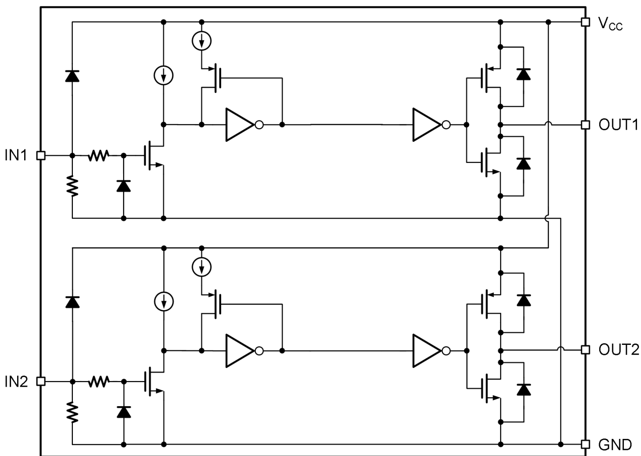
图 10-1 NSG532 功能框图
