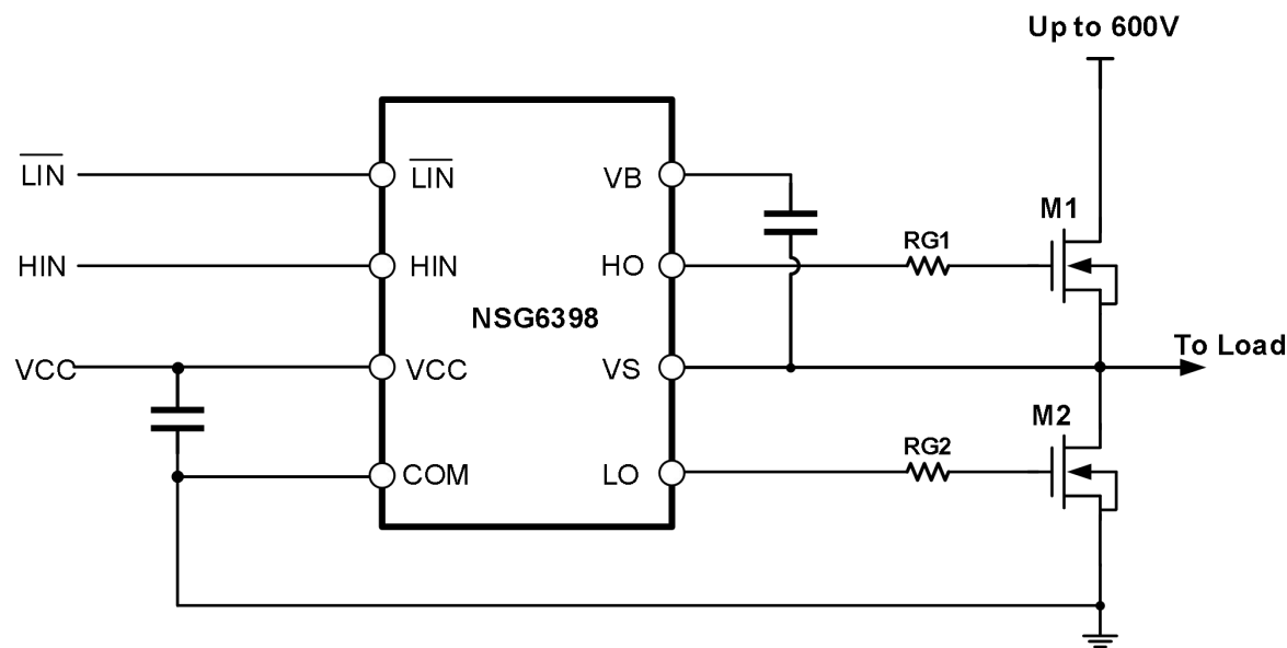
图 10-2 NSG6398 典型应用电路图
