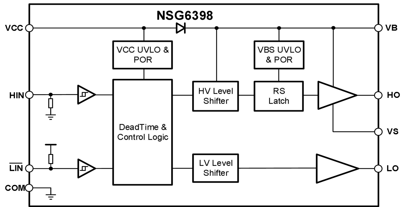
图 10-1 NSG6398 的功能框图
