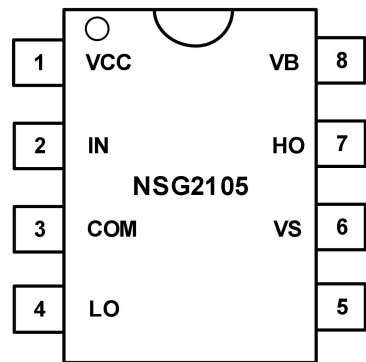
图 7-1 8-脚 SOP8 顶视图
