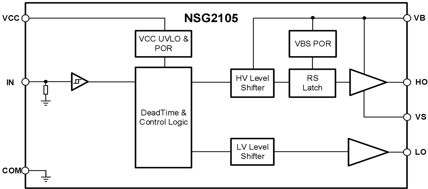
图 10-1 NSG2105 的功能框图
