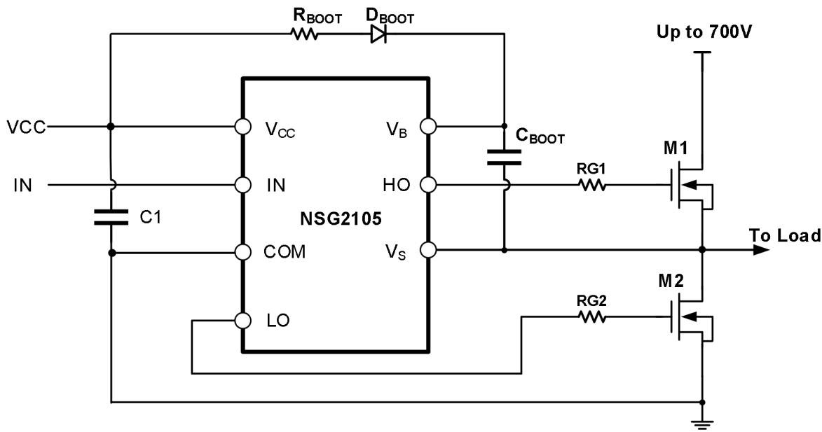
图 10-2 NSG2105 典型应用电路图
