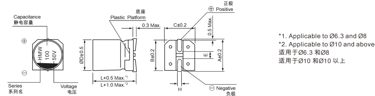
DRAWING 外形图 (Unit: mm)
