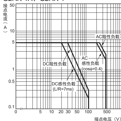
G2RK-1A、G2RK-1
