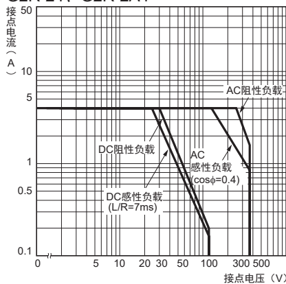
G2R-24、G2R-2A4
