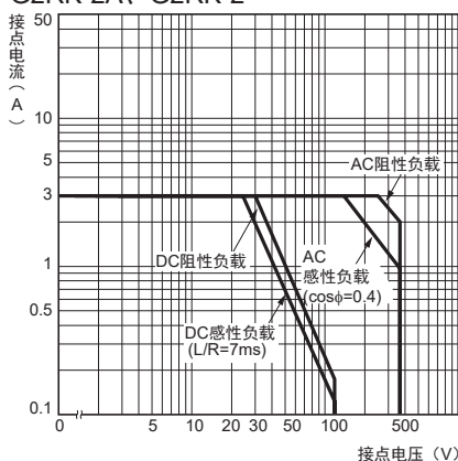
G2RK-2A、G2RK-2
