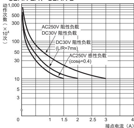
G2RK-2A、G2RK-2
