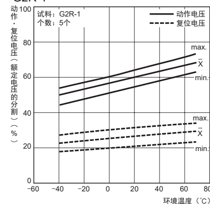
G2R-1
