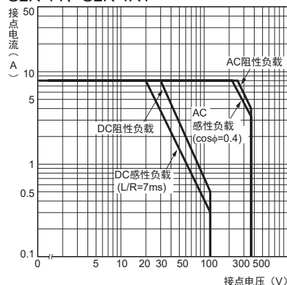
G2R-14、G2R-1A4
