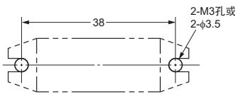
安装孔加工尺寸 (BOTTOM VIEW) 尺寸公差为 \pm 0.1\text{mm}
