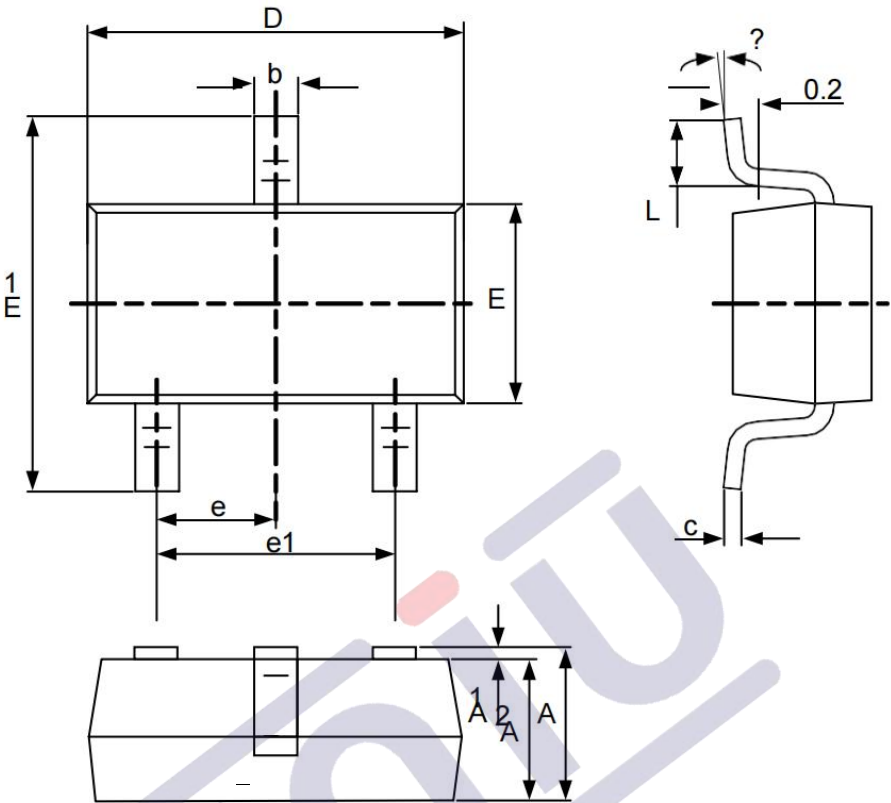
SOT23-3L
