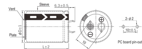
■ 表2 外形尺寸 Dimensions(mm)
