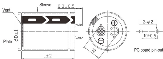
■ 表2 外形尺寸 Dimensions(mm)
