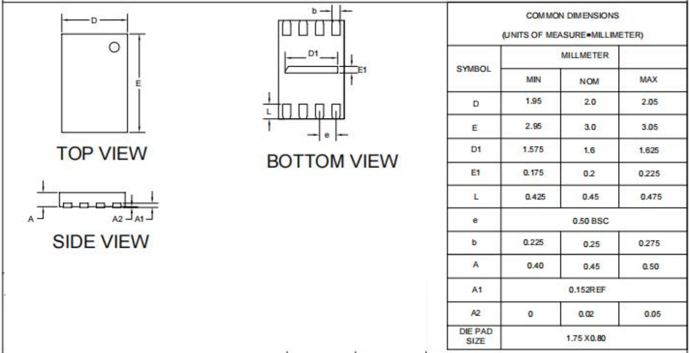
DFN2.0X3.0X0.45-8L产品外形图
