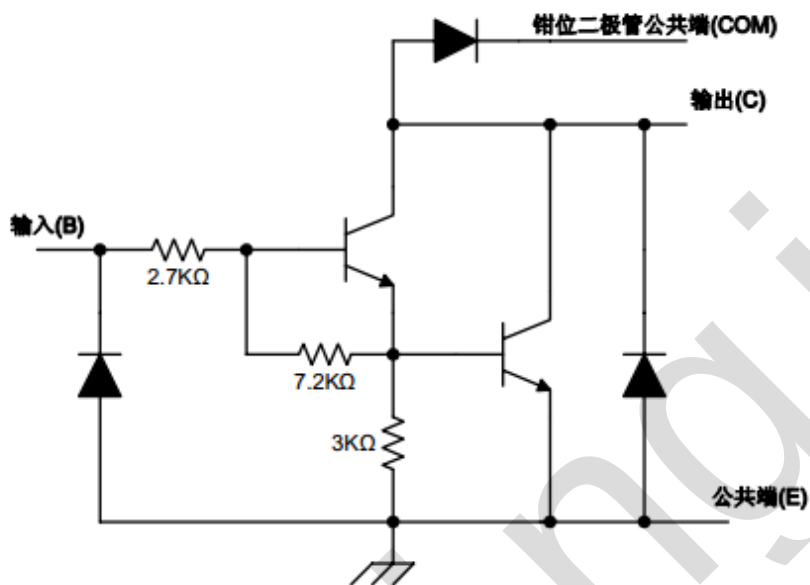
单路驱动电路原理图
