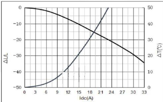
YSPI0740-1R0M
