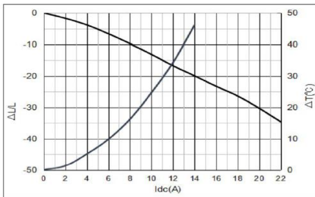
YSPI0740-2R2M
