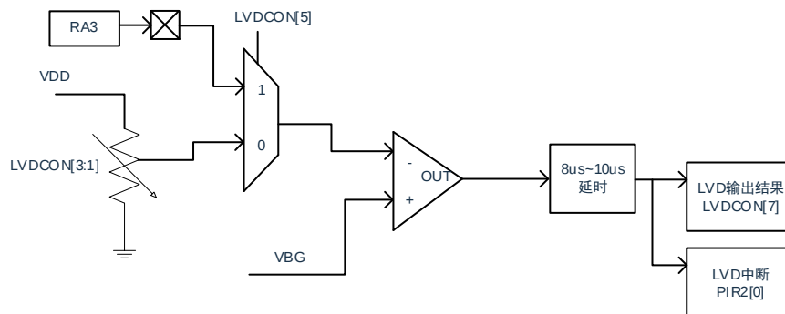
图 16-1: LVD 框图
