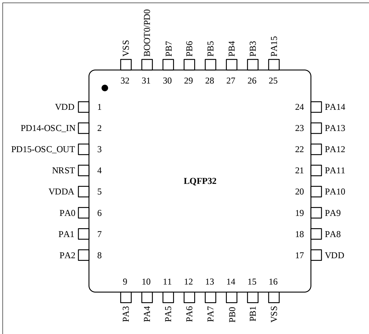
图 3-1 N32L433 系列 LQFP32 引脚分布
