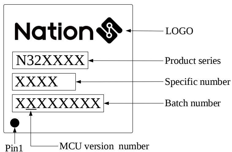
图 5-9 丝印说明
