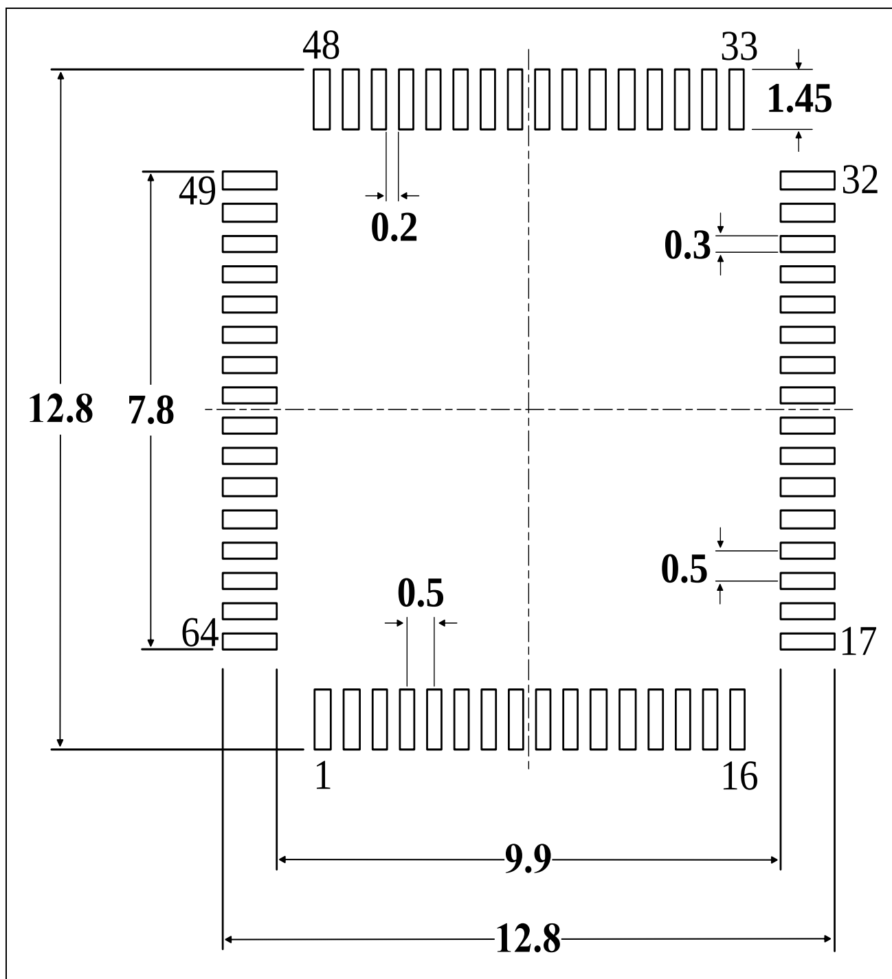
图 5-6 LQFP64 封装焊盘建议 (1)
