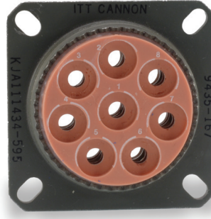
Coax Grommet
