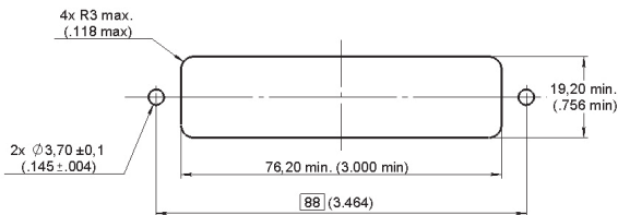
Receptacle
