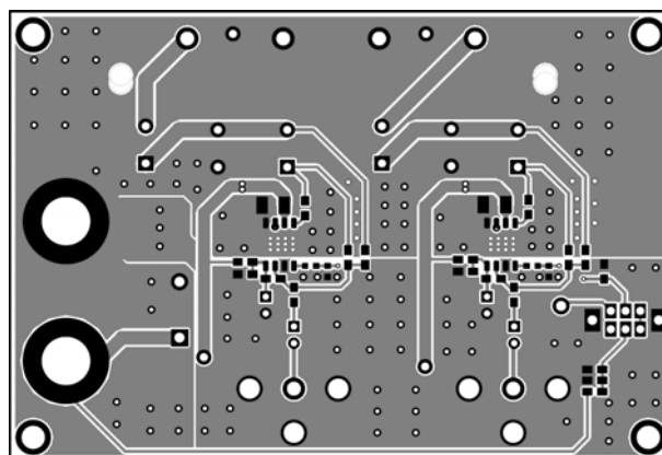
Figure 2—Top Layer
