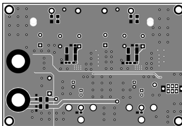
Figure 4—Bottom Layer
