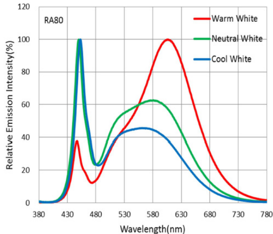
Color Spectrum ( Ra≥80 Tc=25°C)
