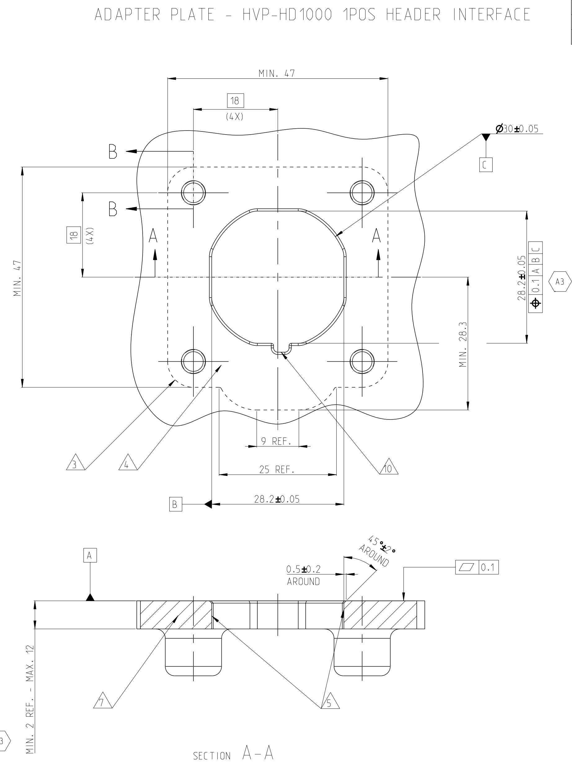
SECTION A-A
