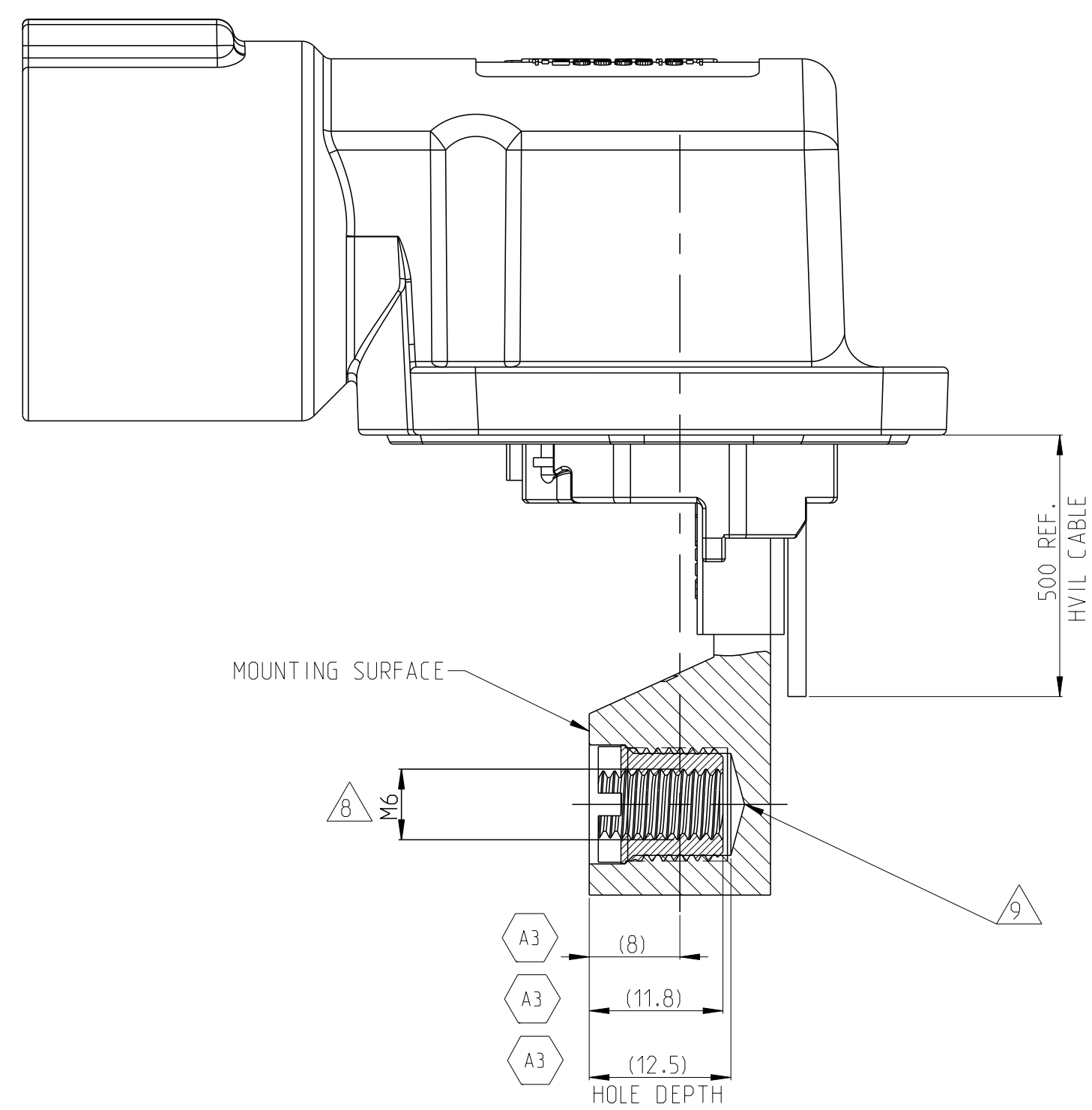
SECTION A-A
