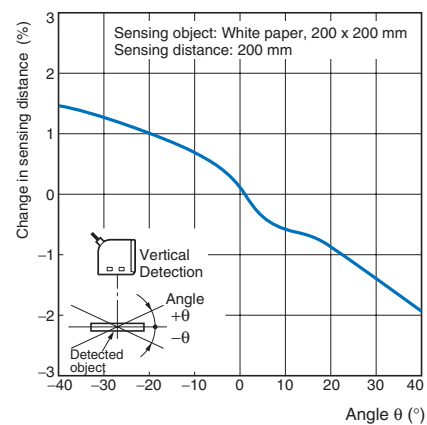
E3S-CL2 Vertical
