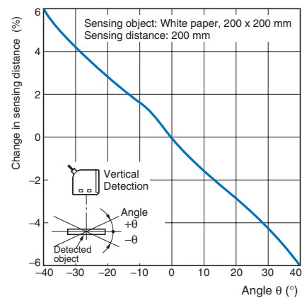
E3S-CL2 Vertical
