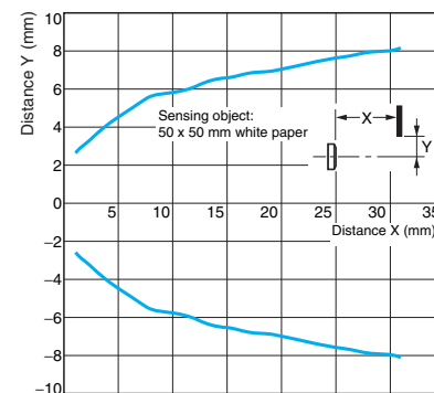
E3T-FL2□
