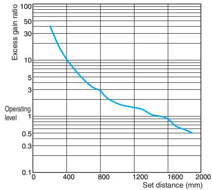
E3T-FT1□F
