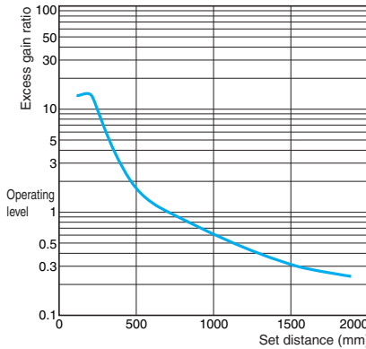
E3T-FT2□F
