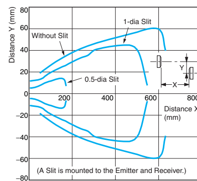
E3T-FT2□F + E39-S64
