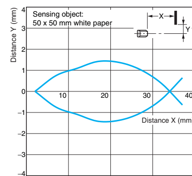
E3T-SL2□(M)
