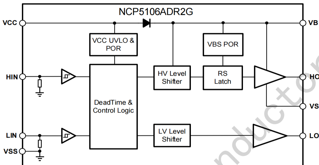
图 7-1 NCP5106A的功能框图
