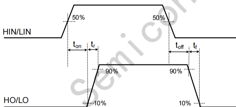
图6-2 输延时波形定义
