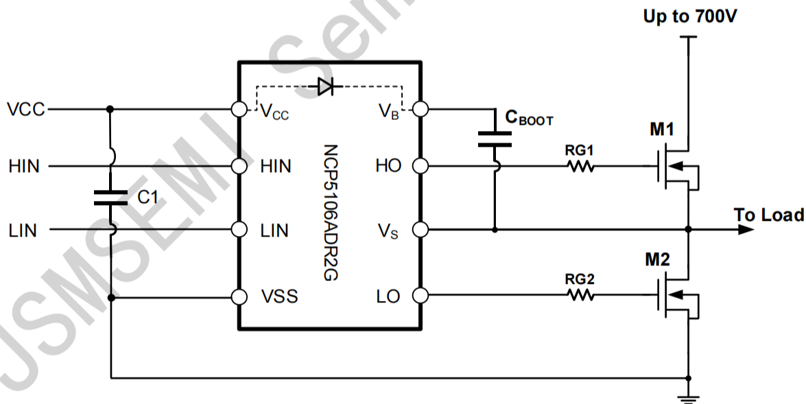
图 7-2 NCP5106A典型应用电路图
