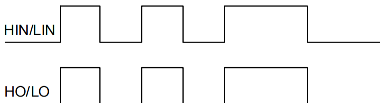
图6-1 NCP5106A 输入输出时序图
