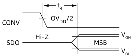
图10. CONV 后启用 SDO ↓
