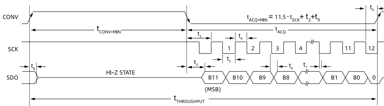
图15. LHA8831 串行接口时序图( t_{\text{CONV}} 期间 SCK 高电平)
