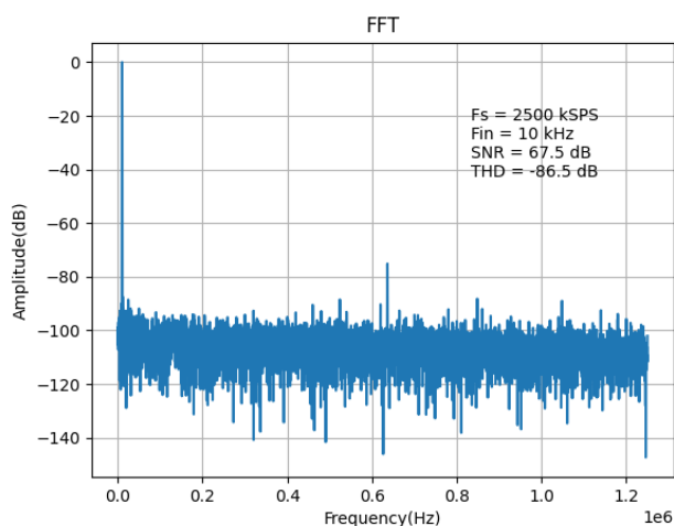
图8. 16k 点 FFT, f_s=2.5\text{Msps} , f_{\text{IN}}=10\text{kHz} , V_{DD}=3.3\text{V}
