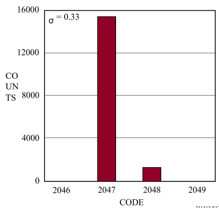
图19. 16384 次转换的直方图
