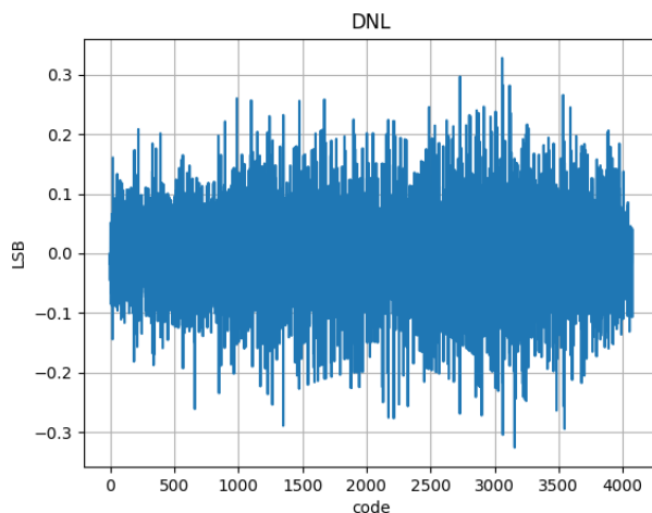
图4. 微分非线性与输出代码, V_{DD}=5\text{V}
