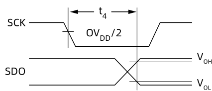
图13. SCK 后 SDO 数据有效访问 ↓
