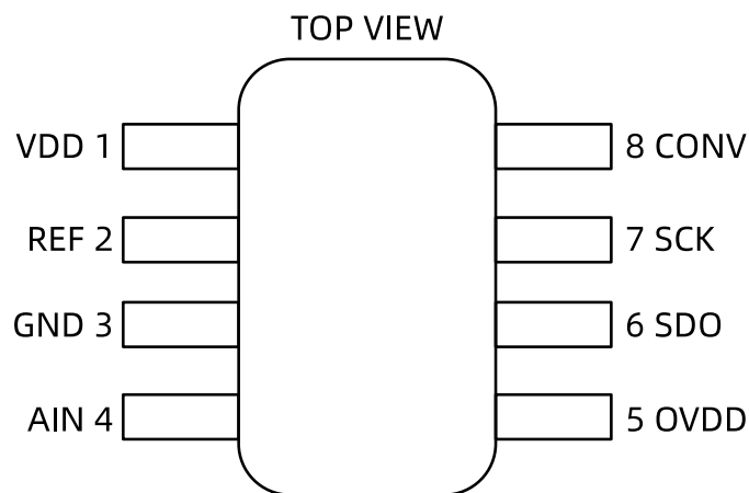
封装 8 引脚塑料 TSOT-23 T_{JMAX} = 150^{\circ}\text{C} , \theta_{JA} = 195^{\circ}\text{C/W} 图2. 引脚配置
