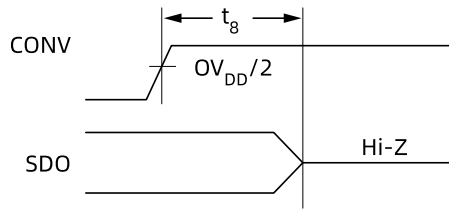
图11. SDO 进入 Hi-Z 后
