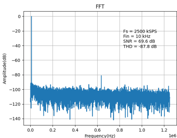
图7. 16k 点 FFT, f_s=2.5\text{Msps} , f_{\text{IN}}=10\text{kHz} , V_{DD}=5\text{V}
