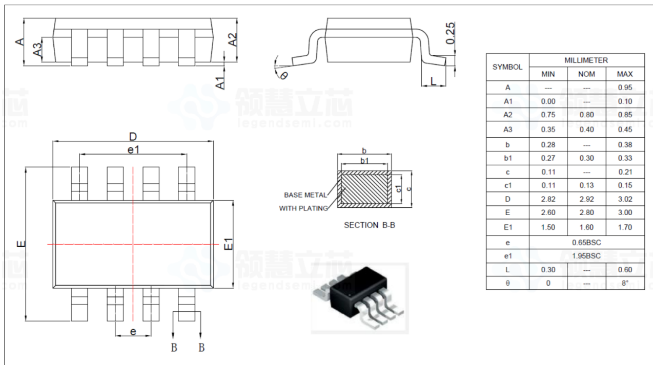
图20. TSOT23-8 封装尺寸图
