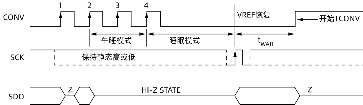
图16. LHA8831 进入退出睡眠模式
