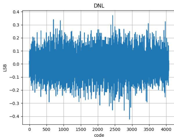
图6. 微分非线性与输出代码, V_{DD}=3.3\text{V}
