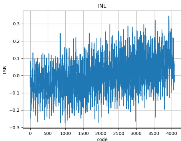
图3. 积分非线性与输出代码, V_{DD}=5\text{V}
