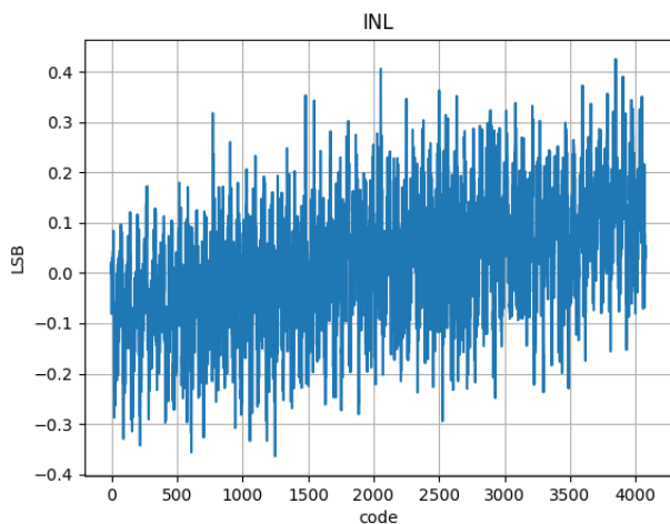
图5. 积分非线性与输出代码, V_{DD}=3.3\text{V}
