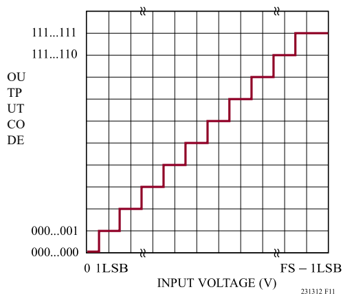
图18. LHA8831 传递函数
