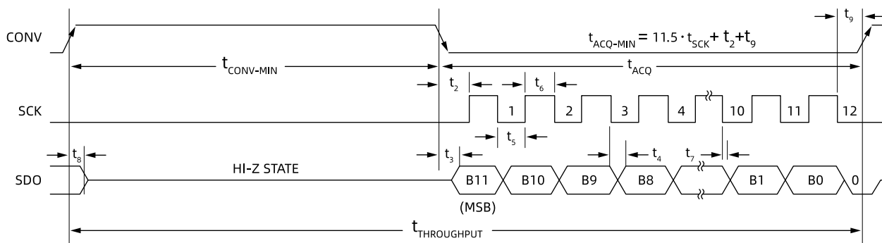
图14. LHA8831 串行接口时序图( t_{\text{CONV}} 期间 SCK 低电平)
