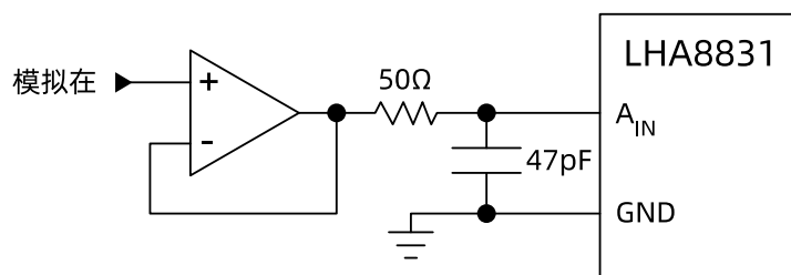
图17. RC 输入滤波器
