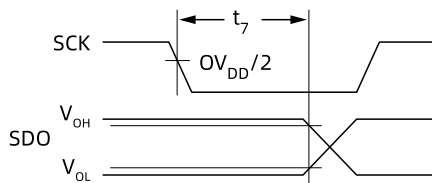
图12. Sdo 数据在 sck ↓ 后有效保持
