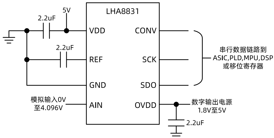
图1. 5V 电源，内部基准，2.5Msps，12 位采样 ADC
