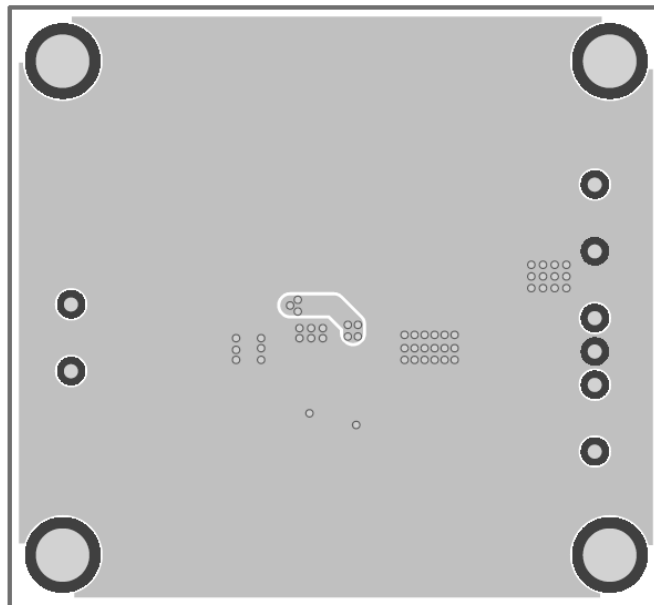
Figure 2—Bottom Layer
