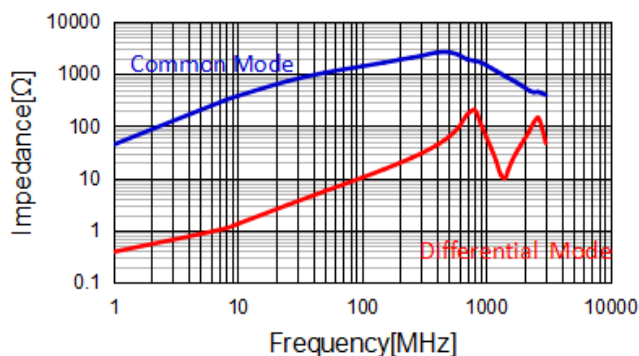
WBA1206D222PT-HF
