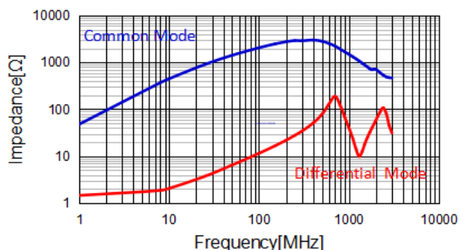
WBA1206D202PT-HF
