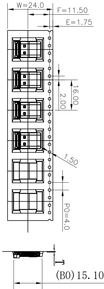
① 产品入载带示意图
