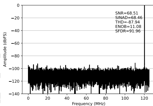
(d) 输入信号频率 = 120MHz
