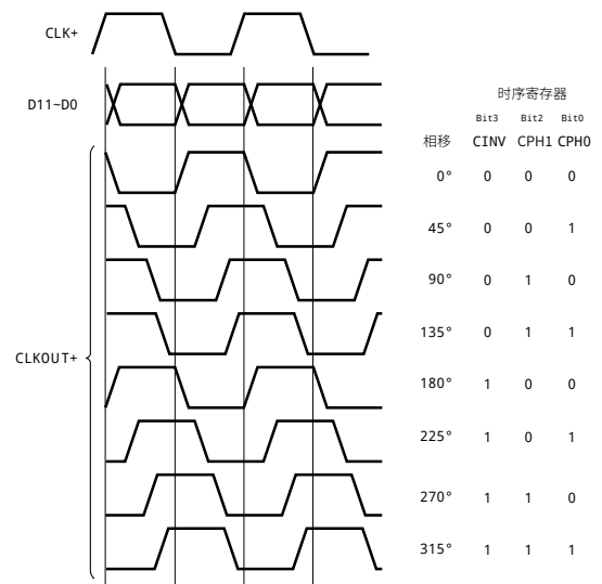
图 13: 相位偏移
