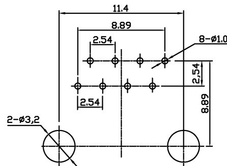
PCB参考图
