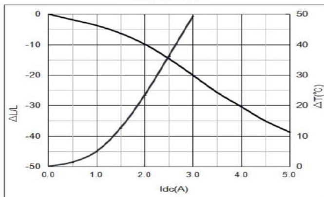
YSPI0850-470M
