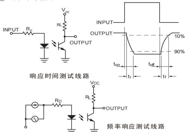
Fig.1 测试线路图
