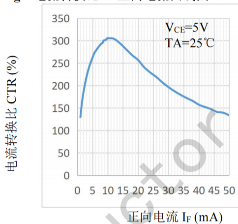
Fig.1 电流转换比 vs 正向电流曲线图
