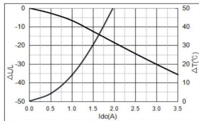
YSPI0850-101M
