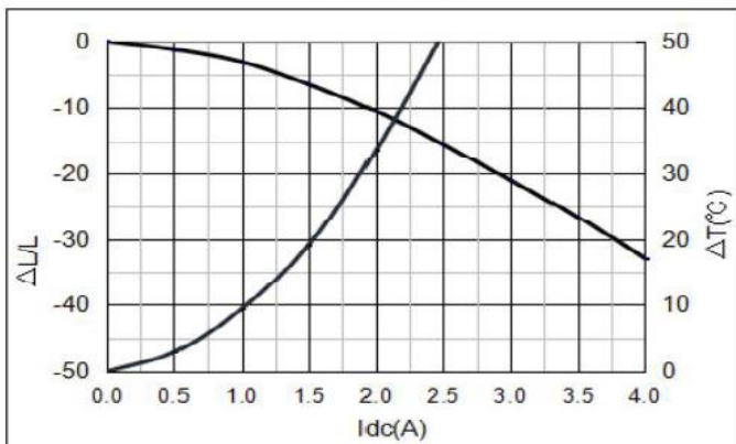
YSPI0850-330M
