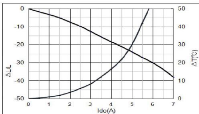
YSPI0850-330M
