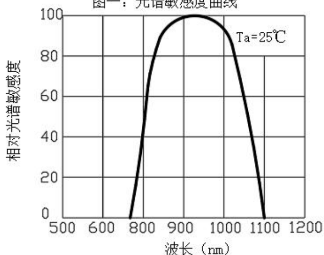
图一：光谱敏感度曲线
