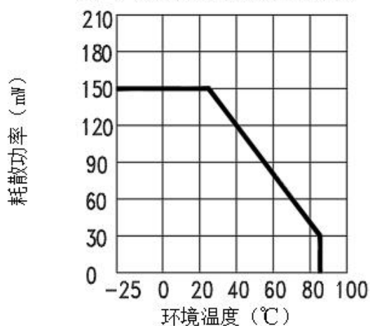
图三：耗散功率VS环境温度曲线
