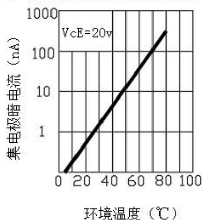
图二：集电极暗电流VS环境温度曲线
