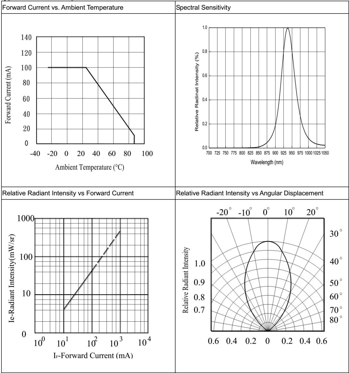
IR 光电特性图 Typical Characteristics For IR
