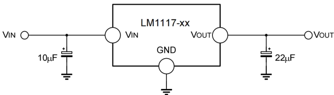
图 1. 典型固定输出电压
