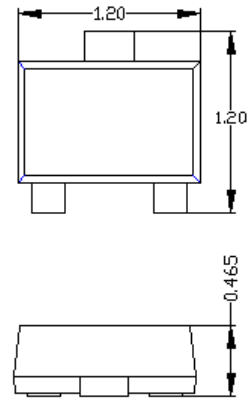
SOT723
