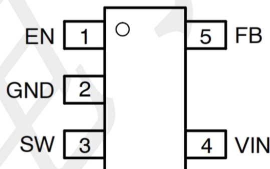
SOT23-5
