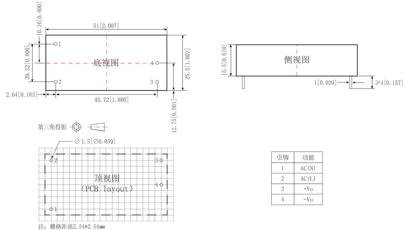
标准式封装
