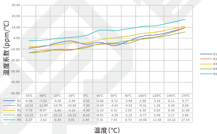
SEWF3951系列0.8mΩ温度系数实测数据表
