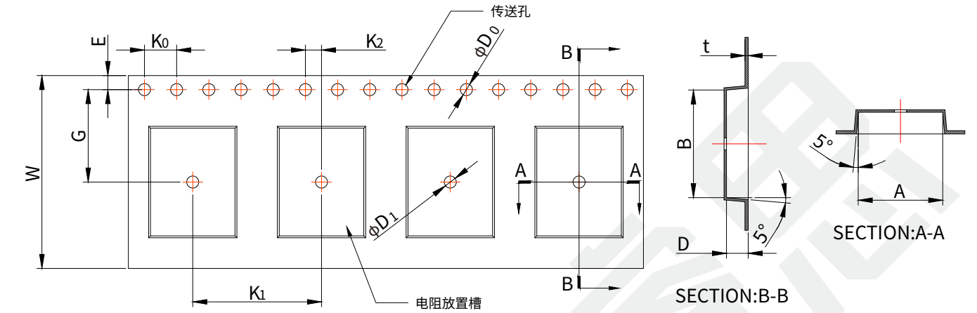
卷编带尺寸图
