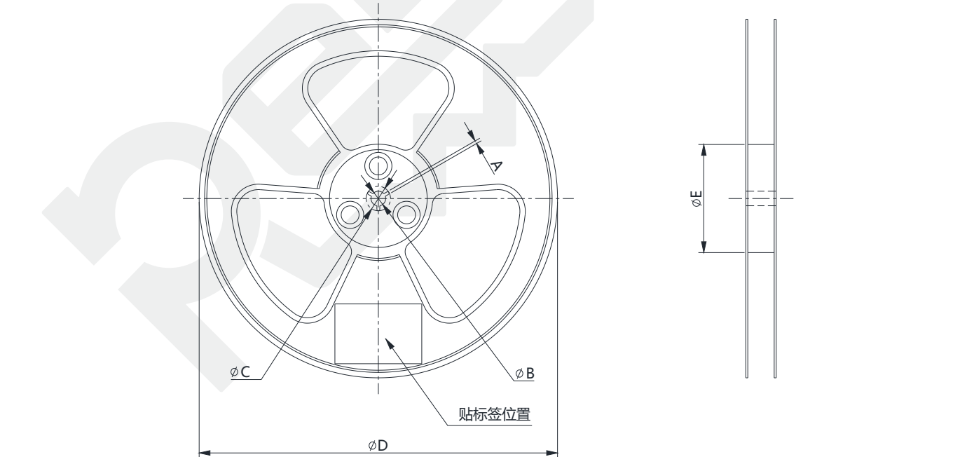
卡盘尺寸图
