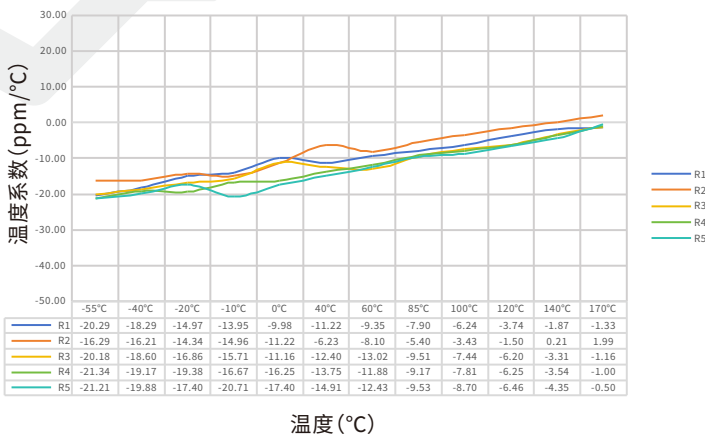
SEWF3951系列0.4mΩ温度系数实测数据表
