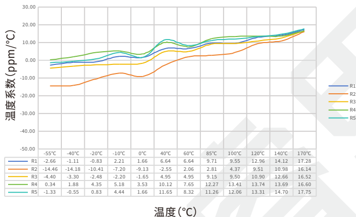
SEWF3951系列0.3mΩ温度系数实测数据表
