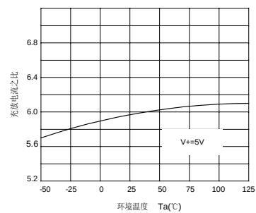
充放电电流之比与温度关系
