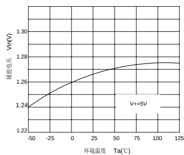
峰值电压与温度关系
