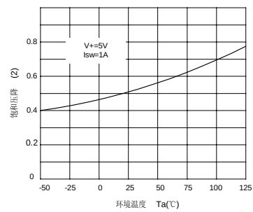
饱和压降 (2) 与温度关系
