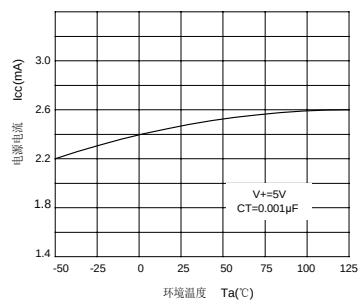
电源电流与温度关系
