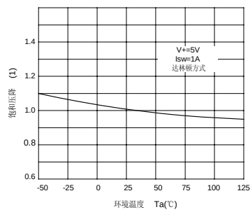
饱和压降 (1) 与温度关系
