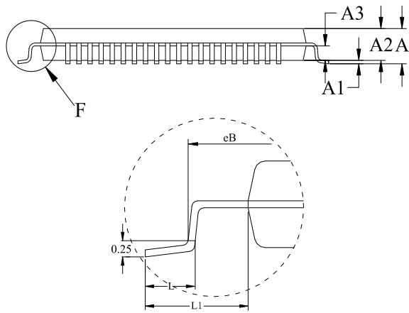
DETAIL: F
