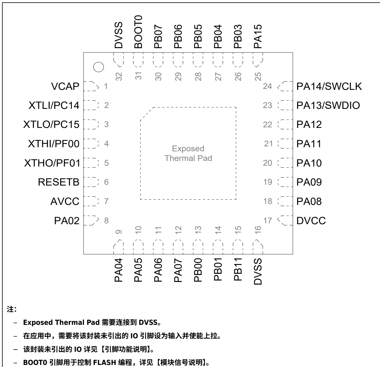
图 3-1 引脚配置图
