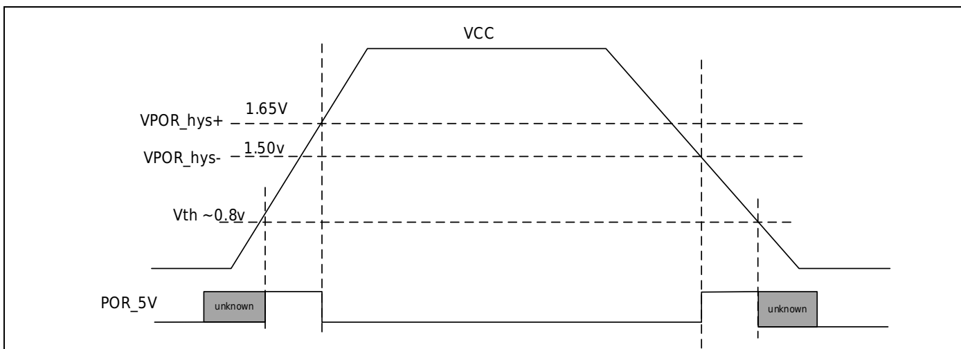
图 7-1 POR/Brown Out 示意图
