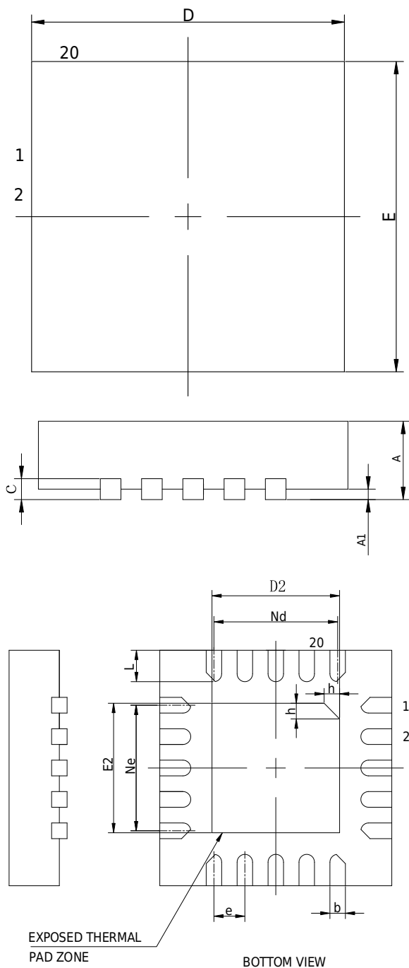
QFN20 封装
