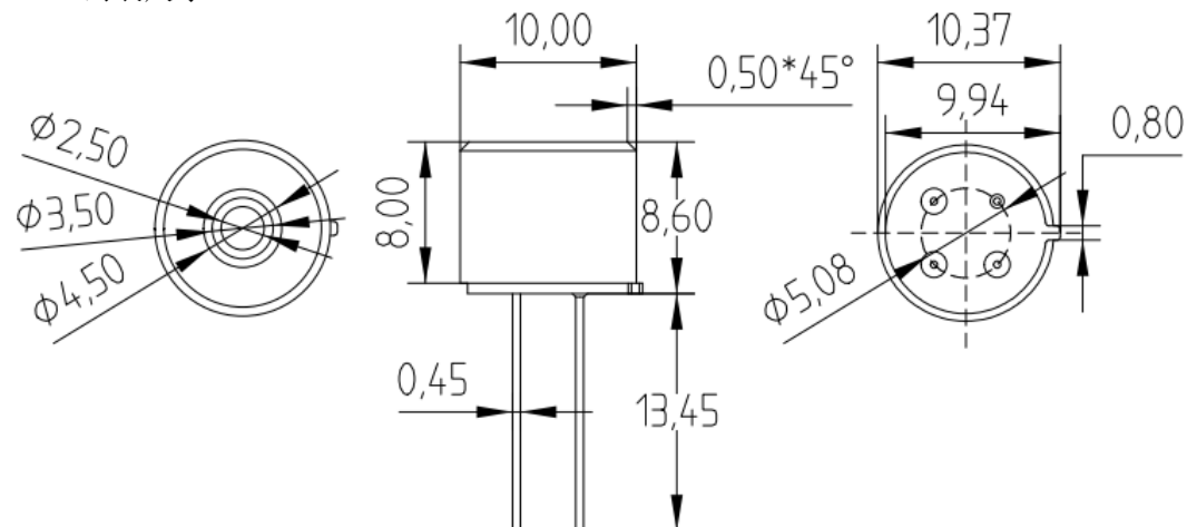
SY-TP-36BPDG-B封装尺寸
