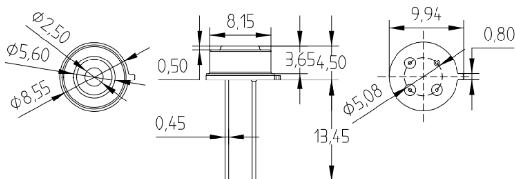
SY-TP-36BPDG-A封装尺寸
