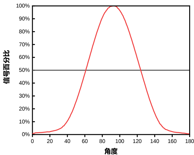
SY-TP-36BPDG视场角
