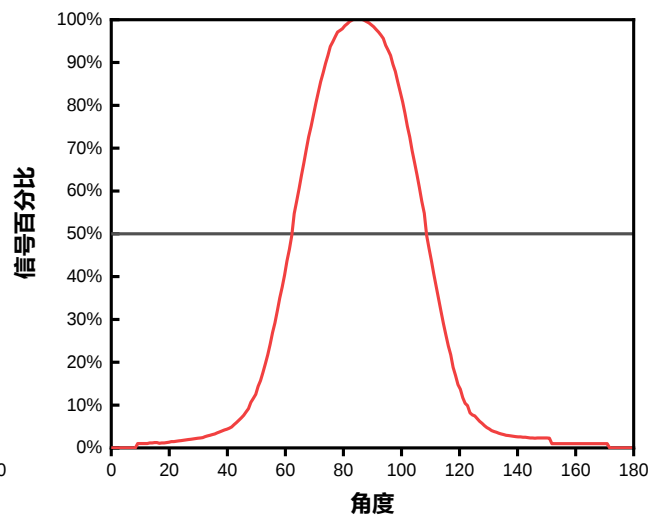
SY-TP-36BPDG-A视场角
