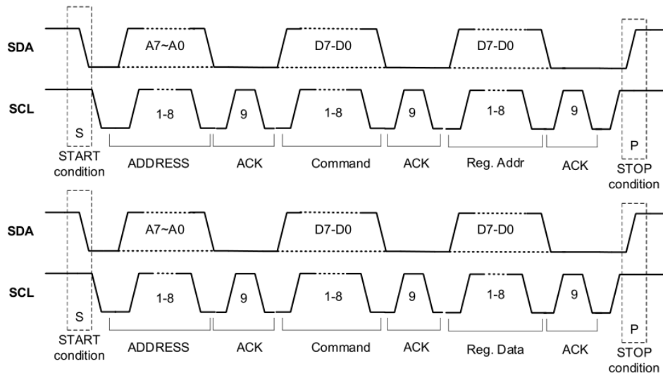
图3：命令模式数据包写入
