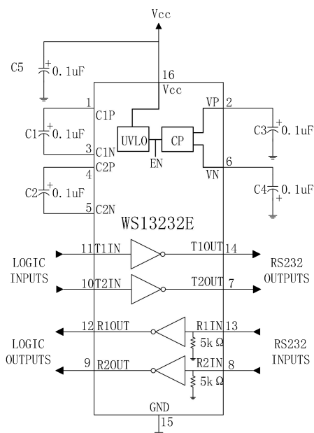
图 6 WS13232E 典型外围应用电路
