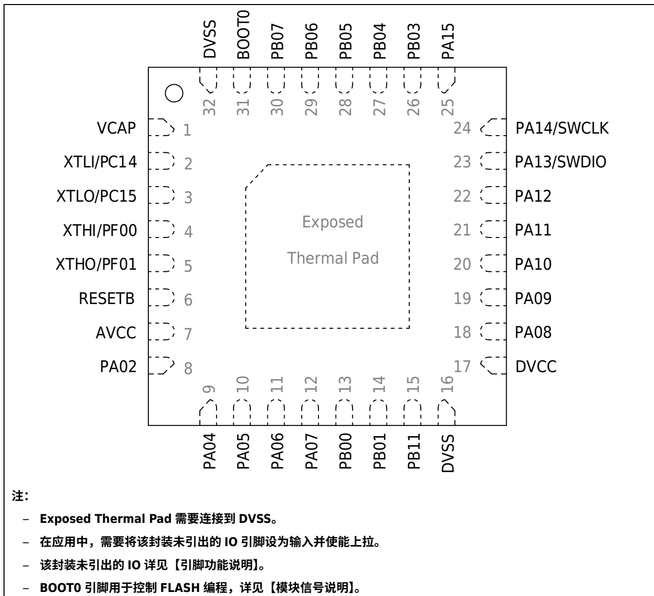
图 3-1 引脚配置图
