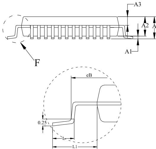
DETAIL: F
