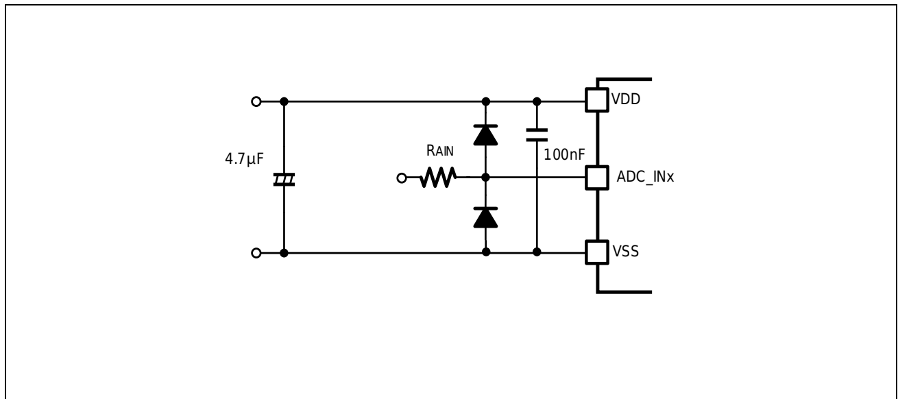
图 3-15 电源和参考电源去耦
