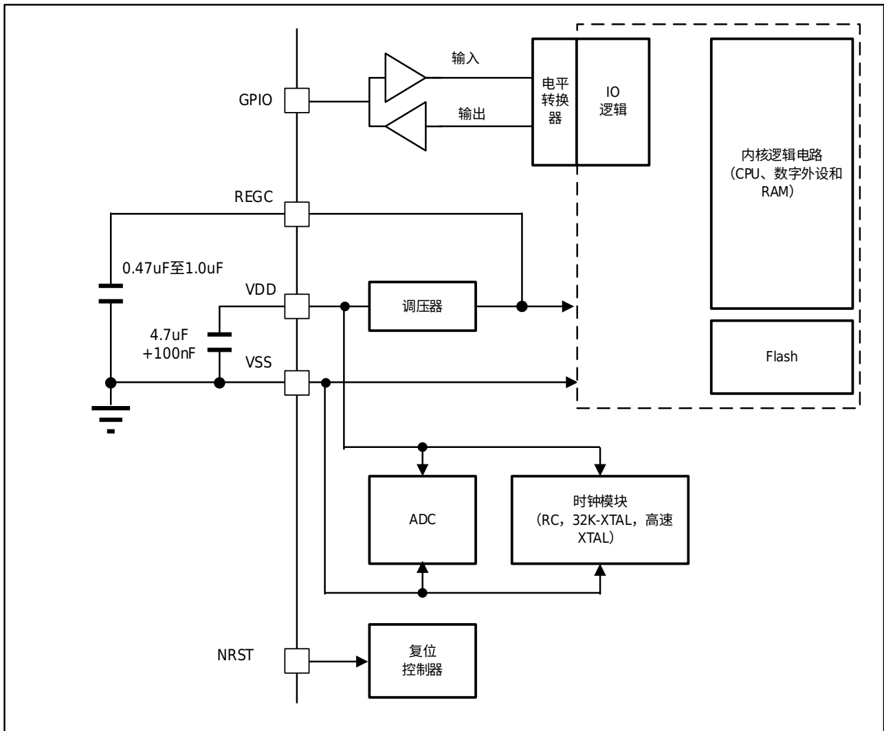
图 3-2 电源方案
