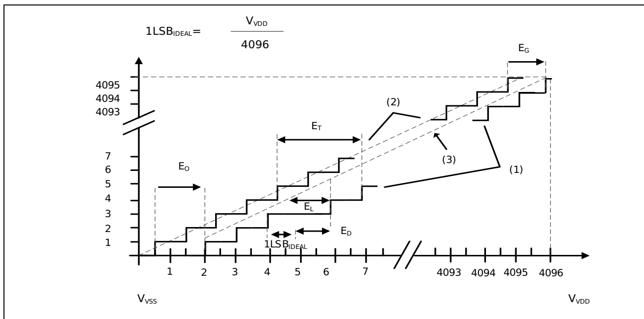
图 3-13 ADC 精度特性
