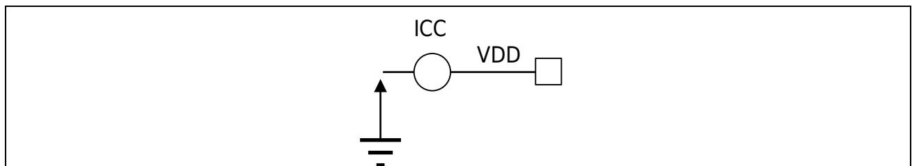
图 3-3 电流消耗测量方案
