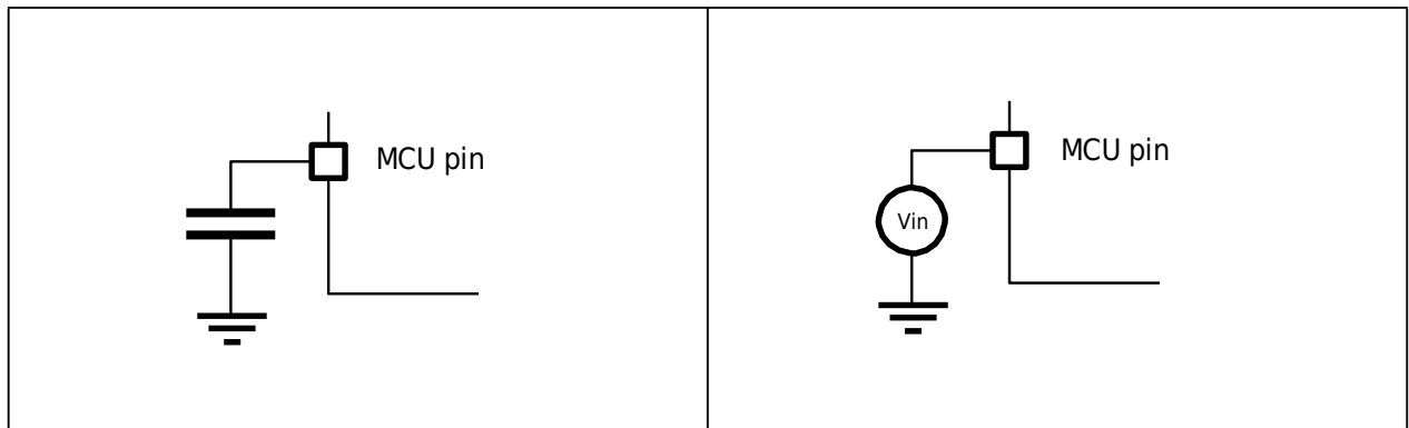
图 3-1 引脚负载条件（左）与输入电压测量（右）
