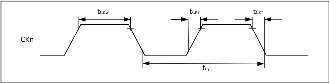
图 3-5 USART 时钟时序
