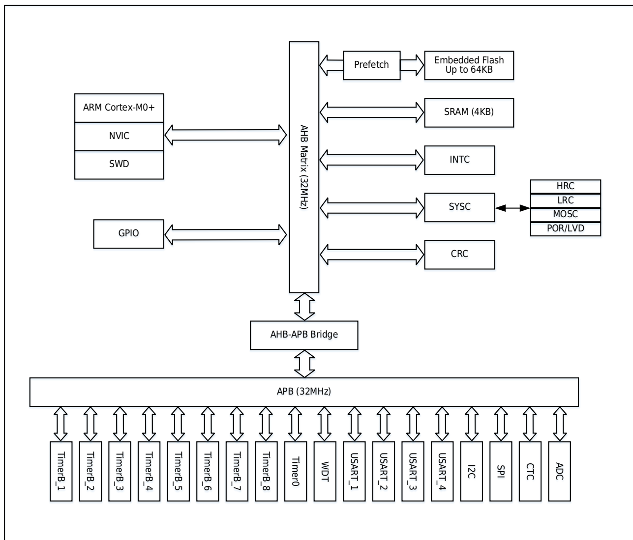
图 1-1 功能框图
