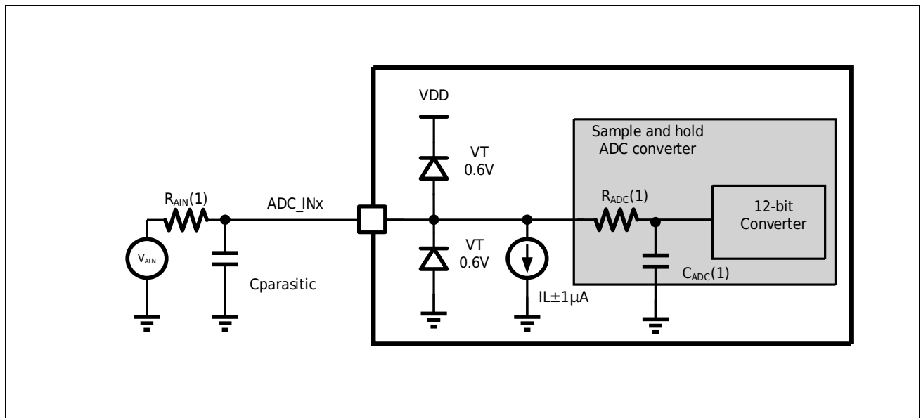
图 3-14 使用 ADC 的典型连接
