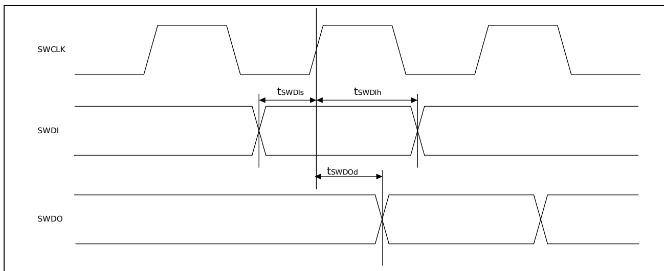
图 3-11 SWDIO 输入输出
