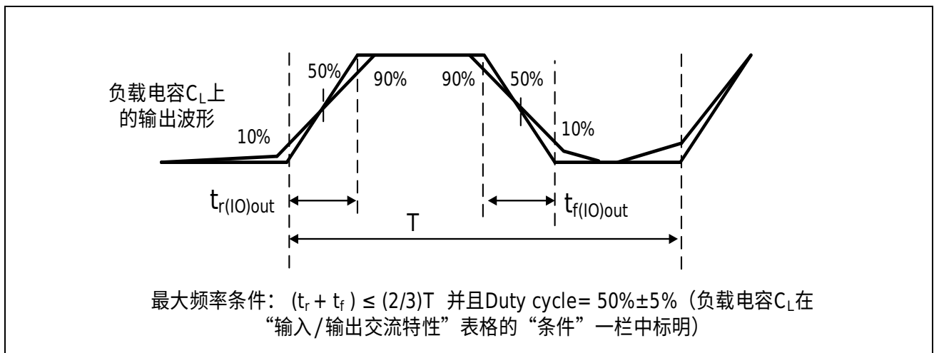
图 3-4 I/O 交流特性定义
