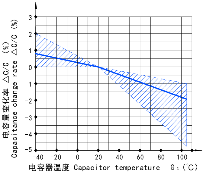
电容量变化率与温度关系曲线图 Capacitance change rate VS capacitor temperature \theta_c
