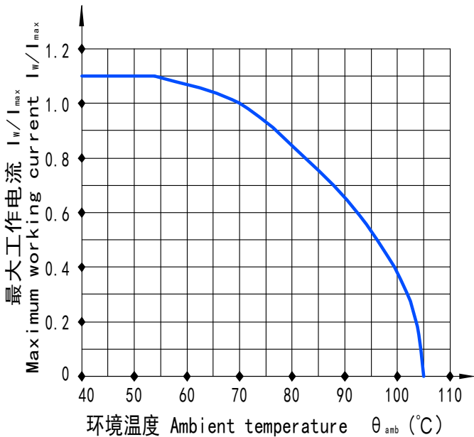
最大工作电流与环境温度关系曲线图 Maximum working current I_w VS ambient temperature \theta_{amb}
