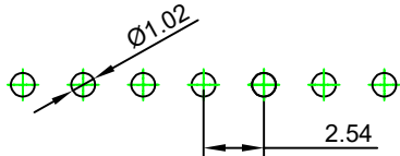
P.C.B Hole Layout
